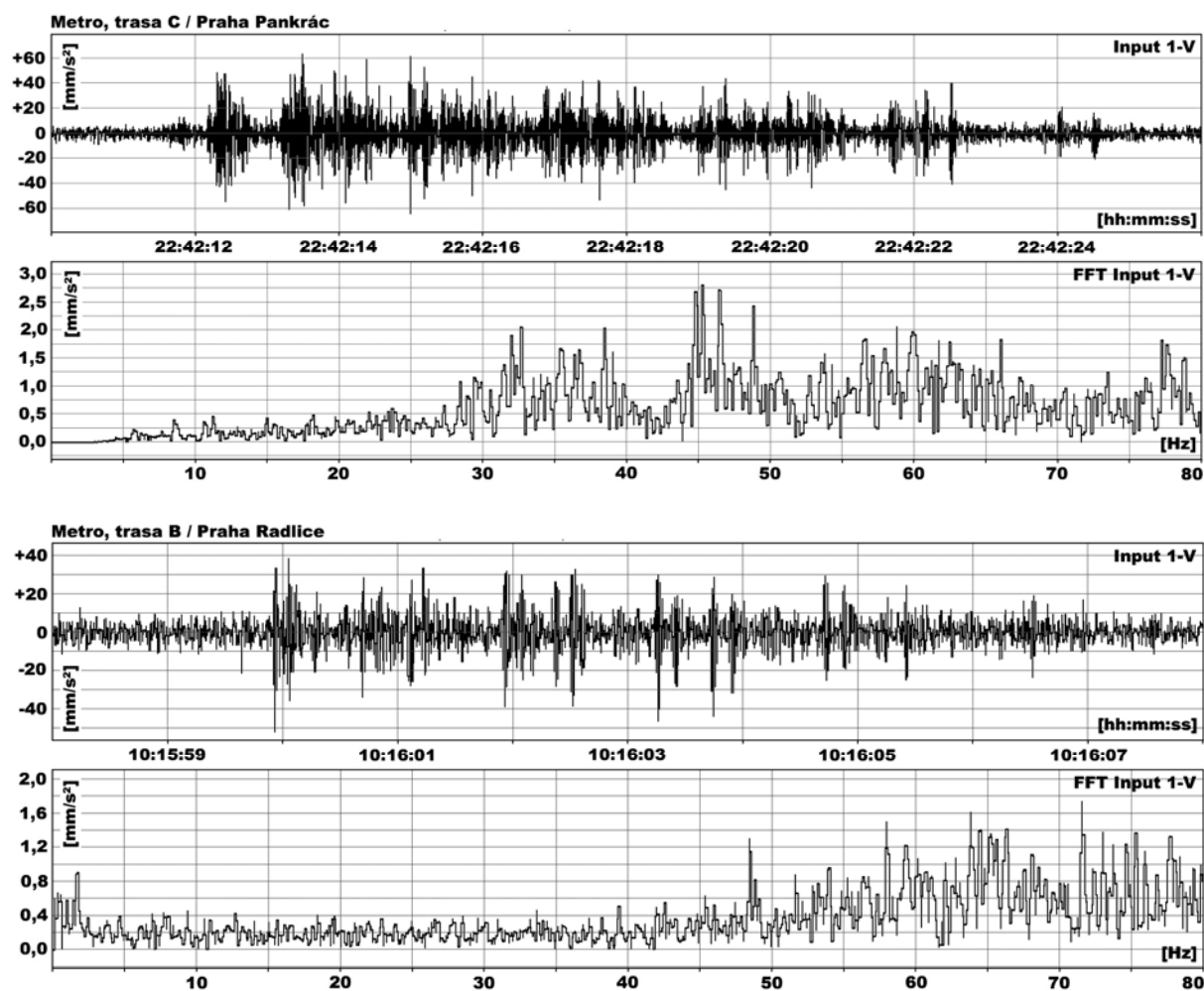
Obr.4 Časové průběhy vertikálních zrychlení a jejich FFT spektra, měřené na konstrukci stanic metra v blízkosti kolejí (Pankrác nahoře, Radlice dole)
